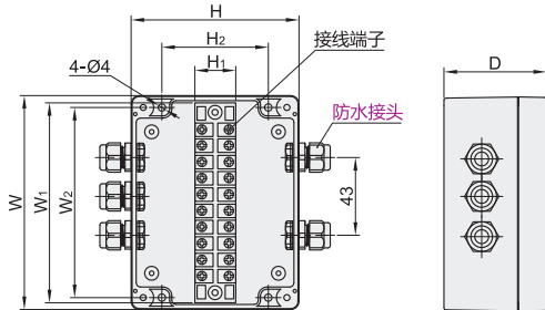
三进二出 ZKN04-3-2-M16
