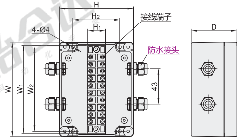
二进二出 ZKN04-2-2-M16
