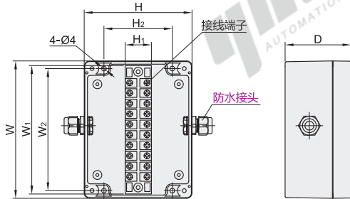
一进一出 ZKN04-1-1-M16
