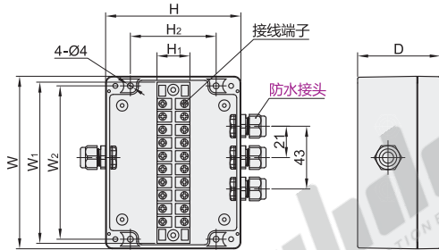
一进三出 ZKN04-1-3-M16
