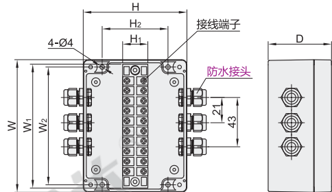
三进三出 ZKN04-3-3-M16
