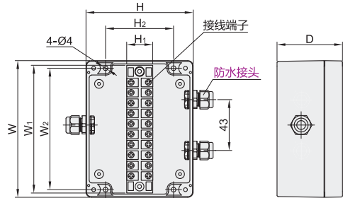
一进二出 ZKN04-1-2-M16
