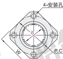
方法兰型
