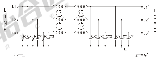
配线图
