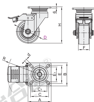
尼龙单刹 J-CPM03
