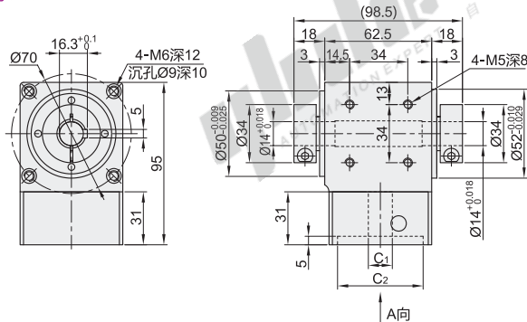
法兰尺寸: 90
