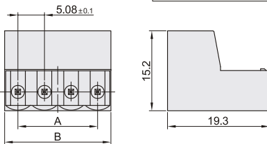
插座 ZKY14
