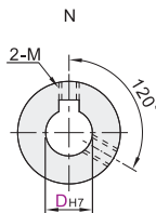
安装方式 (键槽孔型)
