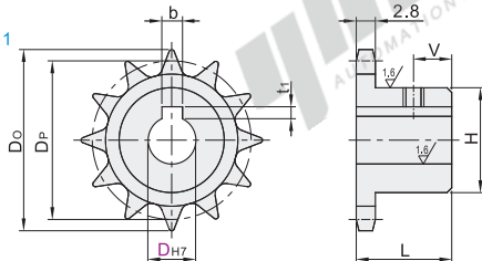
链轮 VLC01/11
