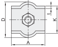
单夹型 TCJ66
