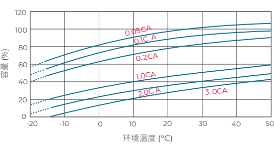
环境温度与放电容量的关系
