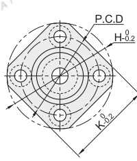
方法兰 E-BFP41/42/46
