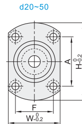
对边法兰 E-BFP51/52/53/54/56
