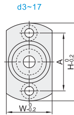
对边法兰 E-BFP51/52/53/54/56
