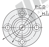
圆法兰 E-BFP31/32/33/34/36
