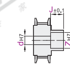
F台阶孔(轮毂侧沉孔)
