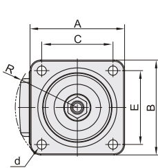
安装面 D60/75
