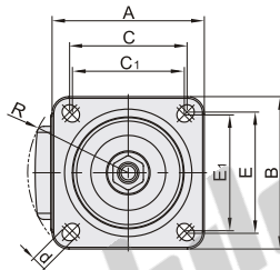
安装面 D60A/75A
