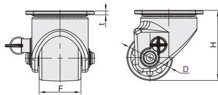
安装面 D60/75
