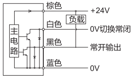
接线图
