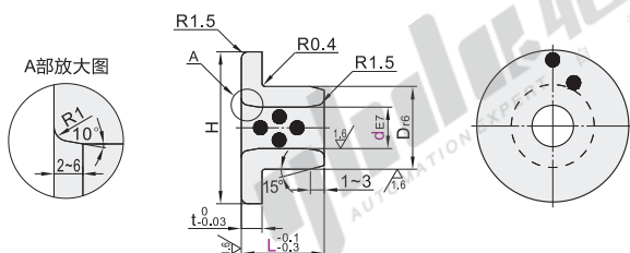
标准型 OFP01
