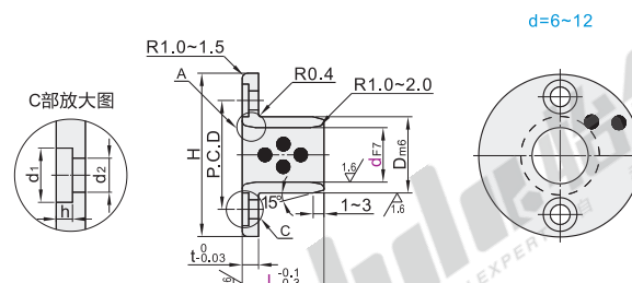
沉孔型 OFP03
