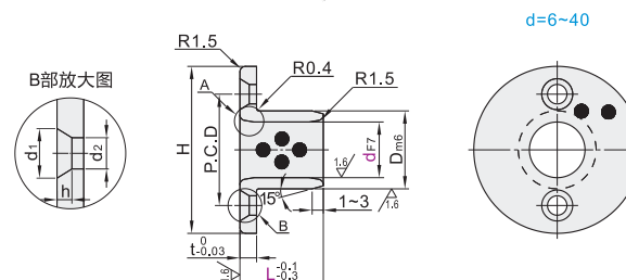
锥孔型 OFP02
