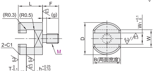
通孔型·外螺纹型 WHN31/32
