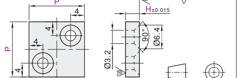
双孔方形 PHR11/12
