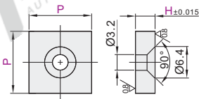
单孔方形 PHR06
