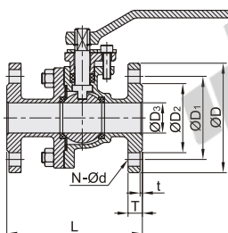
法兰式 BMS80
