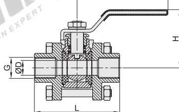
螺纹式 BMS81
