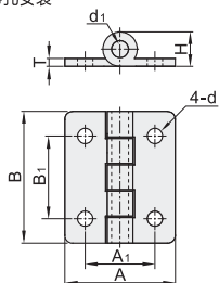
HFV11/12/13/17/E-HFV18/E-HFV19 4孔安装
