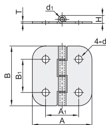
HFV16 4孔安装
