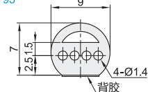
D形带四孔 HGY95
