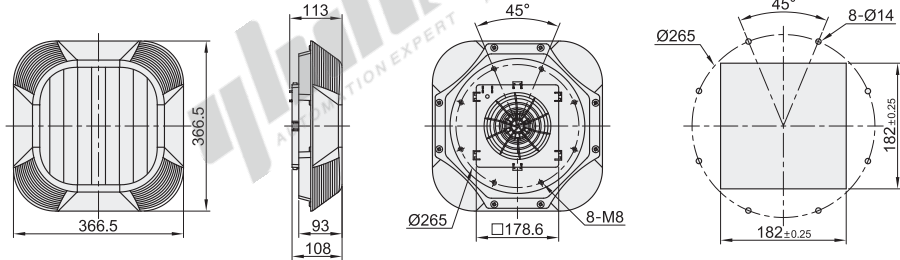
开孔尺寸
