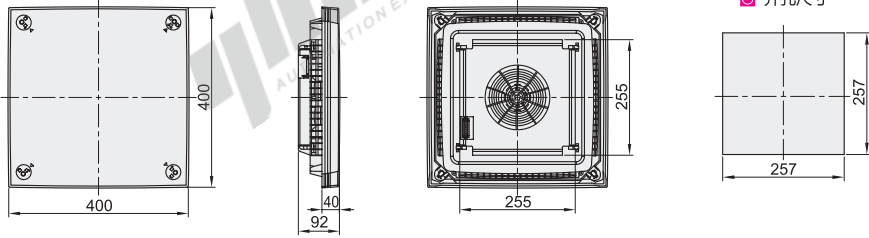
开孔尺寸
