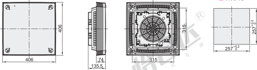
开孔尺寸
