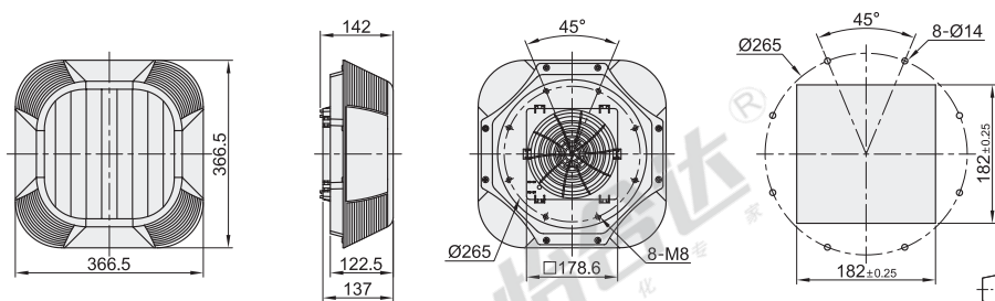
开孔尺寸
