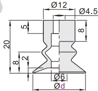
盘径Ø20
