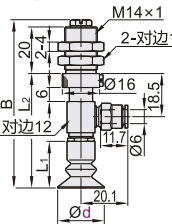
弹簧式侧面真空端口 J-WEU11
