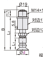
弹簧式直接安装型 J-WEU16
