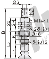
弹簧式顶部真空端口 J-WEU06
