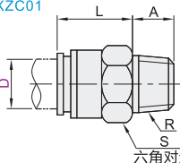
直接头 XZC01
