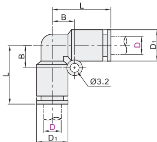
弯接头 XZE11
