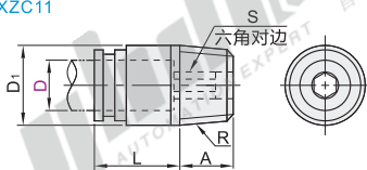
内六角孔直接头 XZC11
