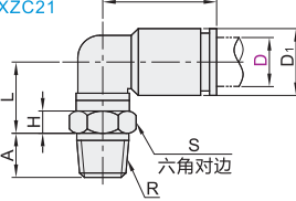
弯接头 XZC21
