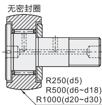
带保持架球面型 BPC25
