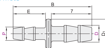
变径 J-XYD92
