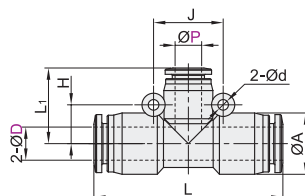
T型三通接头 XZS33
