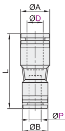
直通接头 XZS31
