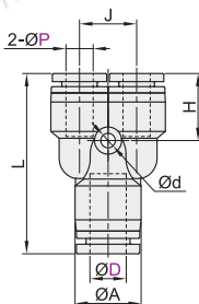
Y型三通接头 XZS32
