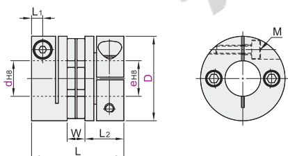
单膜片 DEG03
