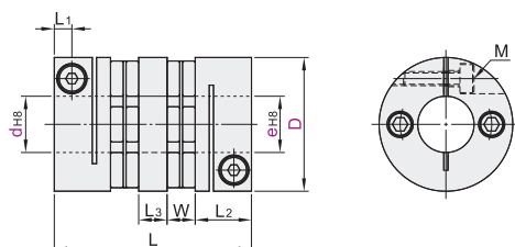
双膜片 DEG13
