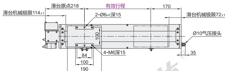
电机安装方式: RD(电机右下折)
