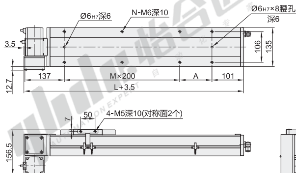
电机安装方式: LD(电机左下折)
