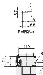
电机安装方式: RD(电机右下折)
