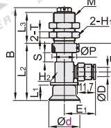
弹簧式侧面真空端口 J-WES71/72
