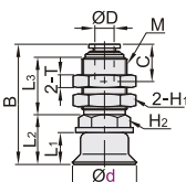
固定式顶部真空端口 J-WES61/62
