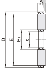
单件 带保持器止推滚针 E-BKL
