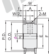
带轮形状：A形
