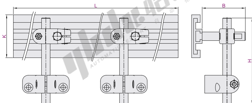
装夹组件+C型护栏组合 ZCE33
