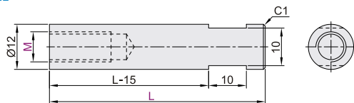
不锈钢内牙杆 ZCE22
