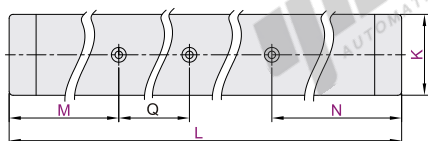
不锈钢钣金 ZCE12
