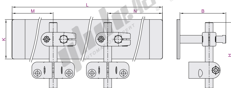
装夹组件+不锈钢钣金组合 ZCE34
