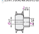
F台阶孔(轮毂侧沉孔)
