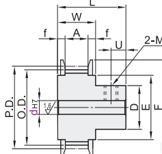
带轮形状: B形
