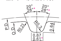
齿形 (ISO标准齿条尺寸)
