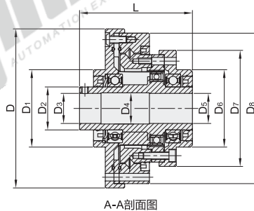
A-A剖面图
