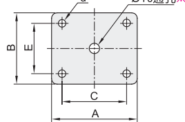
安装面 D75、75A
