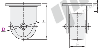
安装面 D75、75A
