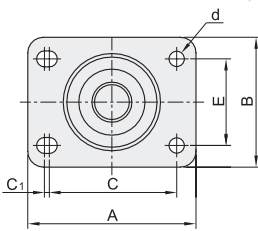
安装面 J-CRB11
