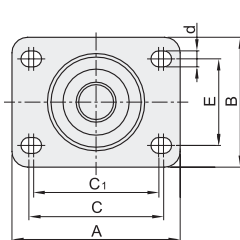
安装面 J-CRB16-D75
