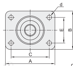
安装面 J-CRB16-D75A/D75B
