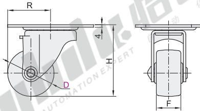
安装面 J-CRB16-D75
