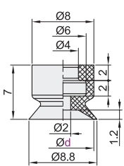
盘径 \varnothing 8
