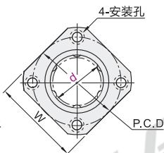
方法兰型 E-LMJ11/12
