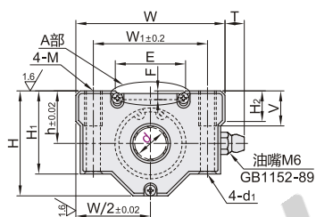
双衬型 LMW59
