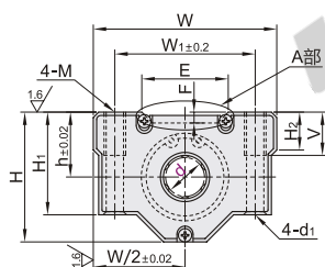
双衬型 LMW59
