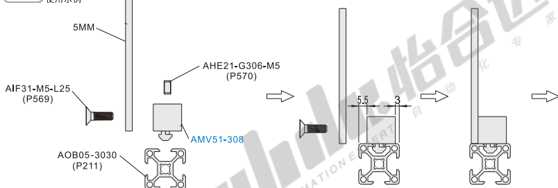
分解图
