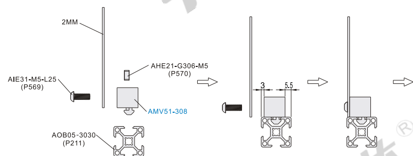
分解图
