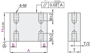
螺纹孔型 PCM21/22/23/25/26/27/28
