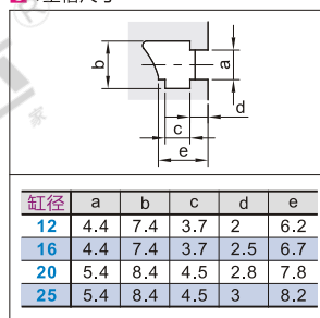
□ T型槽尺寸
