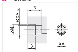
XX部详细图
