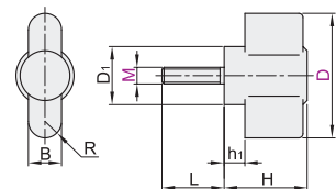
外螺纹型 HAQ11
