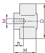
内螺纹型 HAQ16
