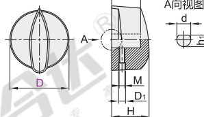
内螺纹型 HAQ17
