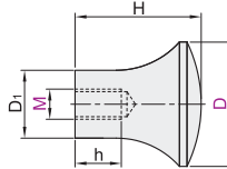
内螺纹型 HAQ07
