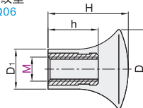
内螺纹型 HAQ06
