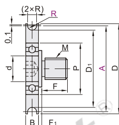
外螺纹型 Y-EKC06/07/08/09
