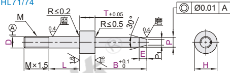
锥角型 YHL31/34 YHL71/74
