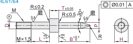
锥头R型 YHL21/24 YHL61/64
