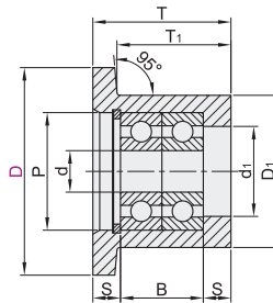
双列轴承 QBR85/86
