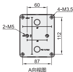
A向视图
