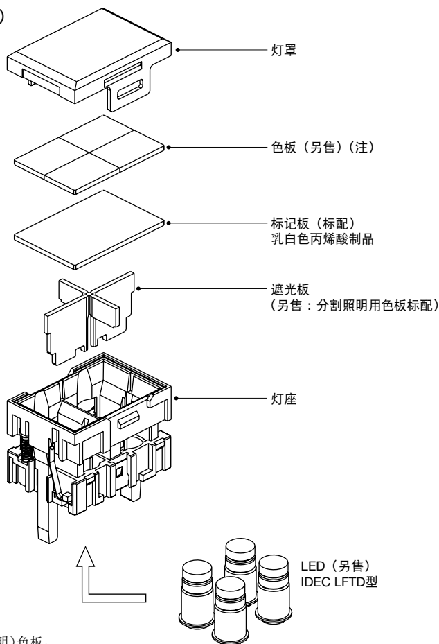
MC3D 型 (全面~4 分割照明)
