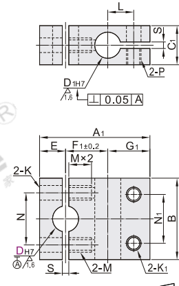
分体式异径正交型 RDL21/22/51/81
