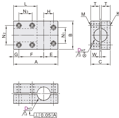
分体式同径T形正交型 RDL01/02/31/61
