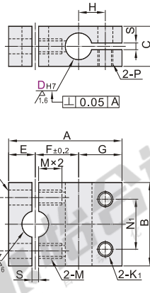
分体式同径正交型 RDL11/12/41/71
