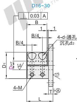
圆法兰型 GAY01/02/06
