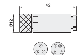
直母头 ZIS46 连接方式: M8
