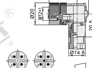
弯母头 ZIS47 连接方式: M12
