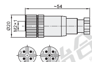
直母头 ZIS46 连接方式: M12
