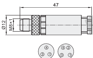
直母头 ZIS46 连接方式: M8
