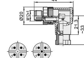
弯母头 ZIS47 连接方式: M12
