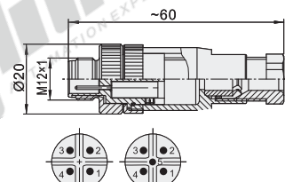
直母头 ZIS46 连接方式: M12
