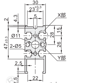
型材截面放大图
